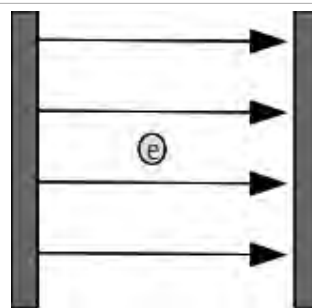
Esquema que representa un electrón dentro de un campo eléctrico.
