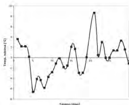
Gráfica de temperatura mínima contra tiempo en la ciudad de Toluca en noviembre de 2010.)
